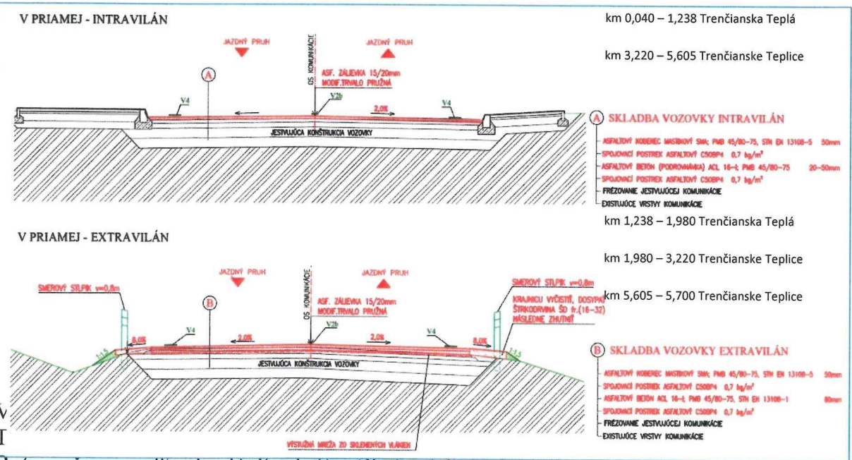
Obrázok č. 1: Porovnanie navrhnutého technického riešenia rekonštrukcie vozovky v intraviláne (A) a extraviláne (B)
